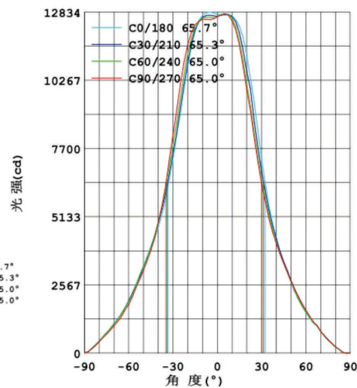
光强分布曲线
